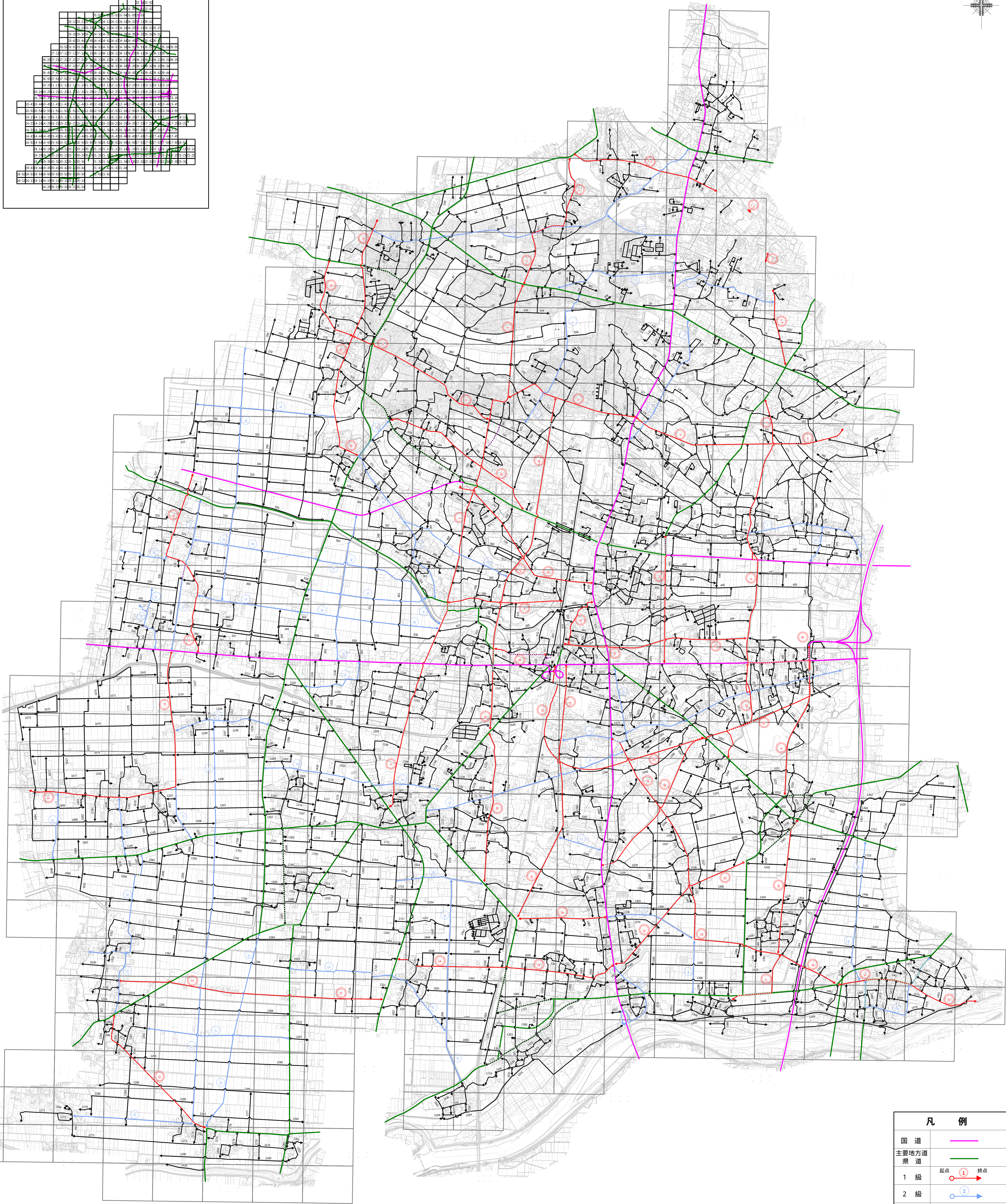
図郭割
