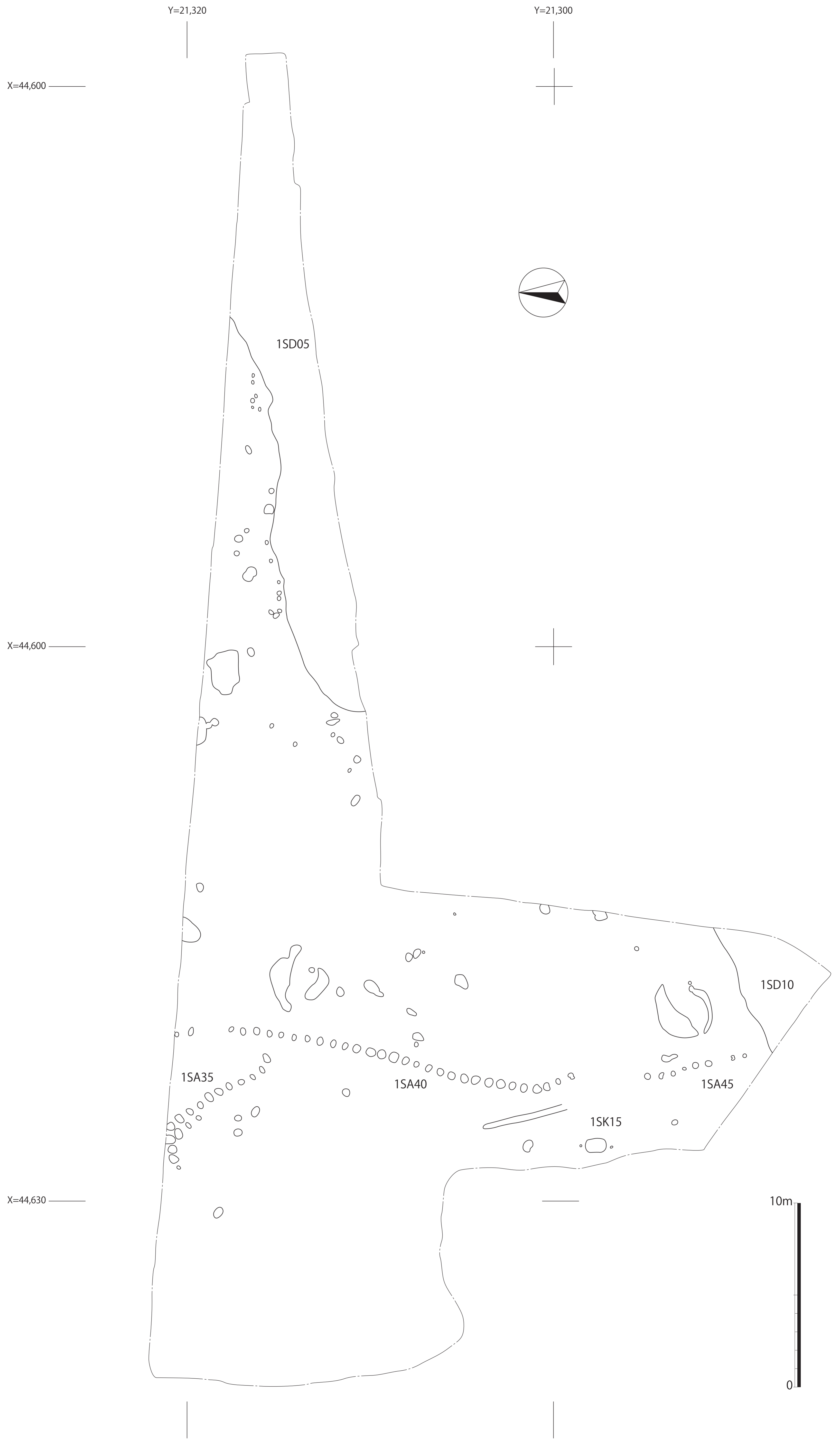
筑後東部地区遺跡群Ⅷ久恵上川原第1次調査【A区】遺構略側図(1/100)
