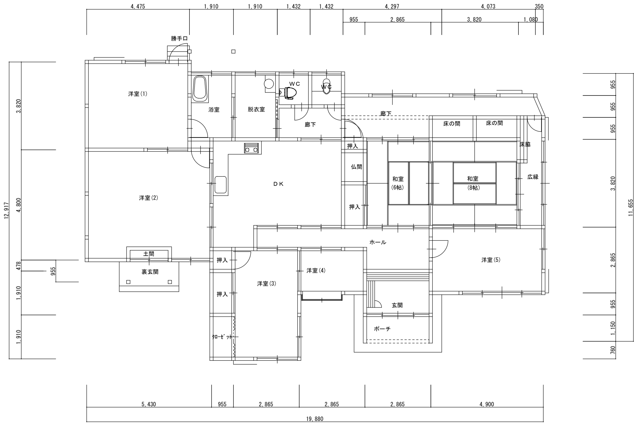
平面図 S=1/100
