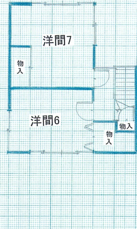
2階平面図
