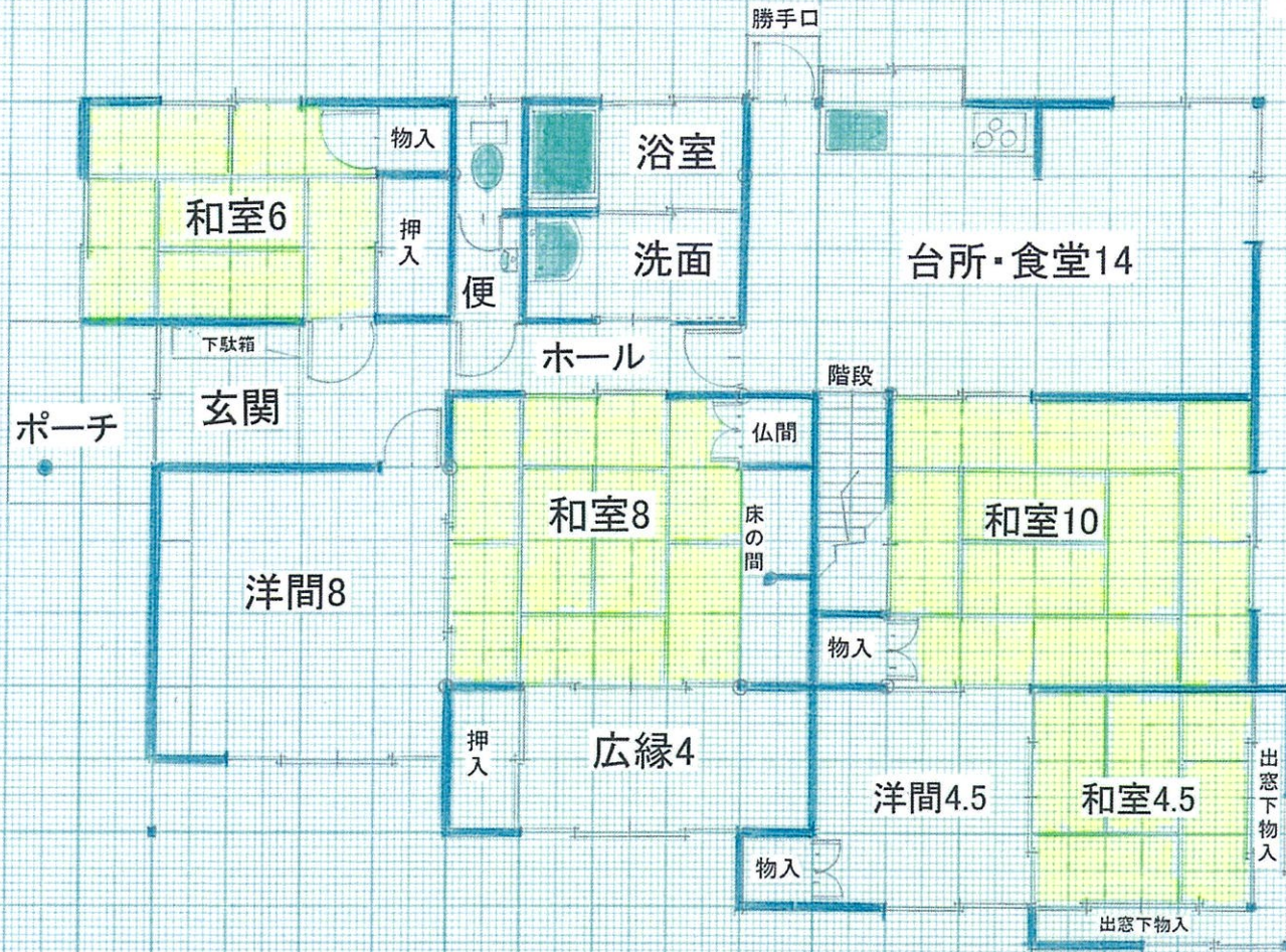
1階平面図
